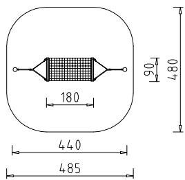
45272 Hängematten-Schaukel, mit Stahlseilnetz und Stahlrohrstehern
