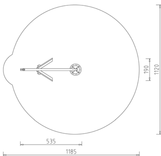
45221 Leimbinder Nest-Pendelschaukel, 4 m hoch
